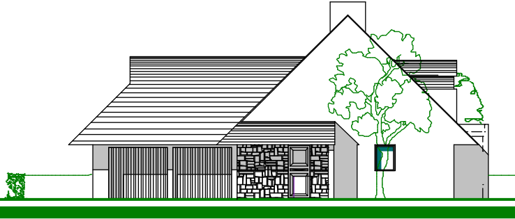
Elévation OUEST
