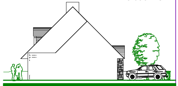
Élévation EST
